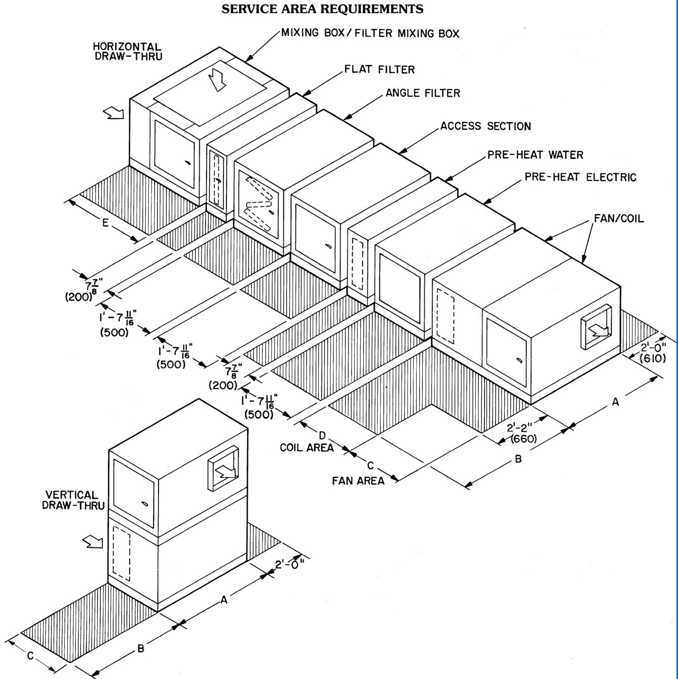
DIMENSIONS (ft-in.)
